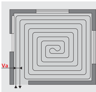
Abbildung 2: Schneckenförmige Rohrführung V_a = Verlegeabstand
